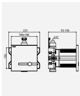
TEMPOMATIC mit dualer Steuerung Batteriebetrieb Art. DELABIE: 464SBOX + 464006
