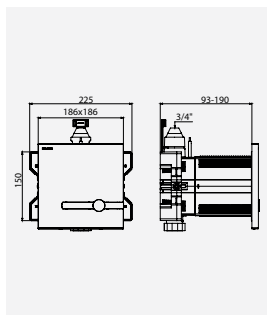
TEMPOMATIC mit dualer Steuerung Netzbetrieb Art. DELABIE: 464SBOX + 464000
